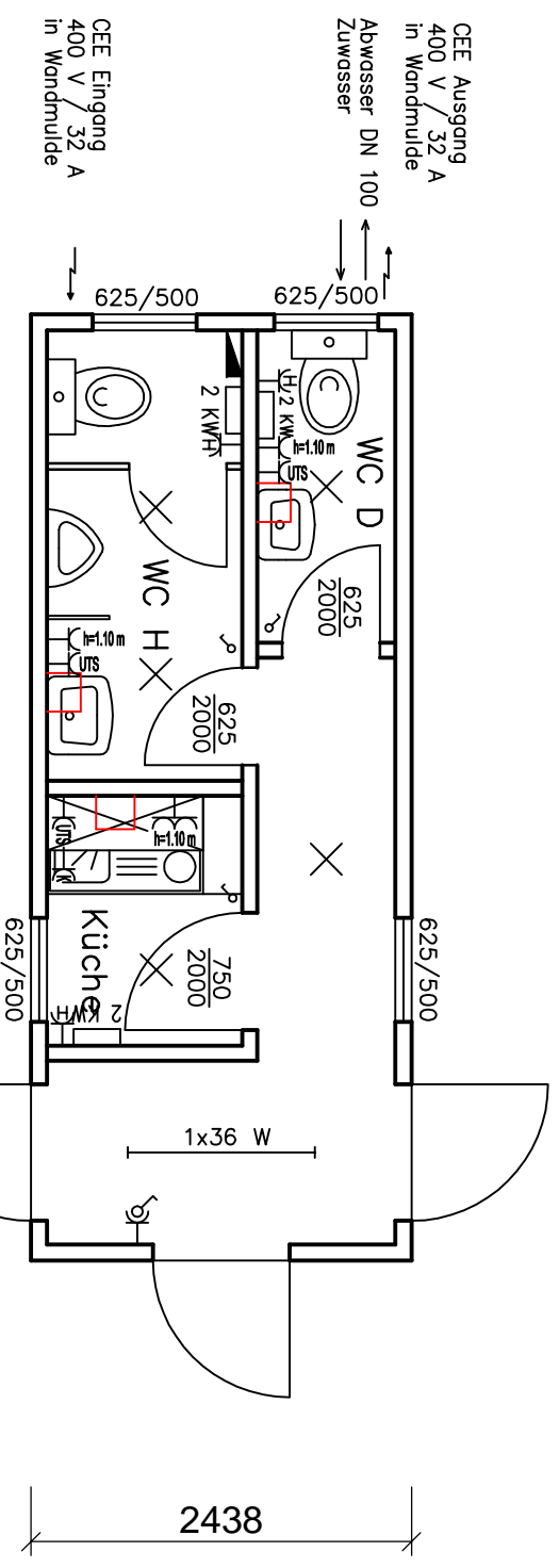
Typ T1 S Kombi
